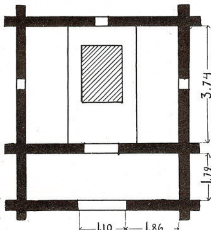
Fig. 9. Bastu. Plan.
